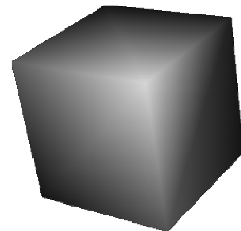
Gouraud shading 51
